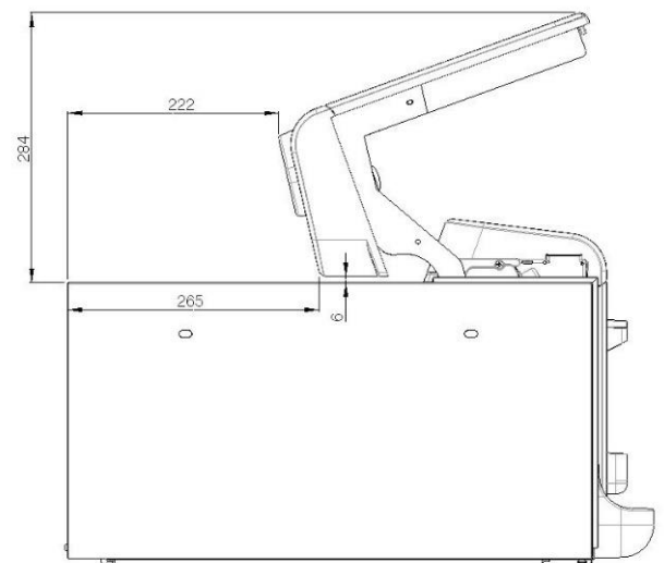
Maximalöffnungswinkel
