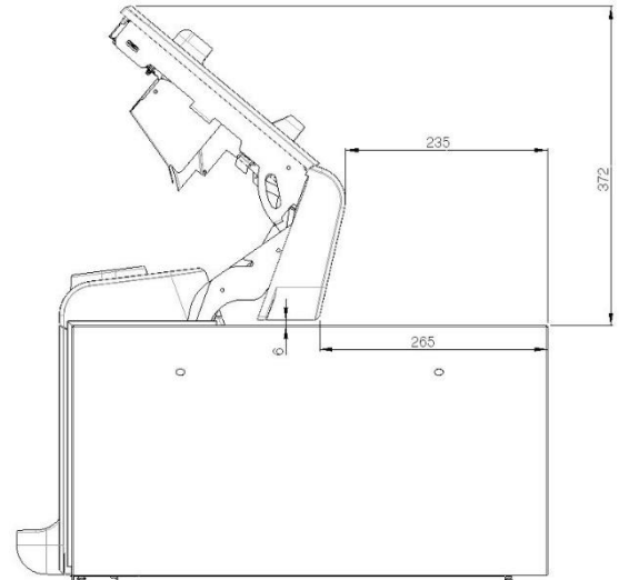
Maximalöffnungswinkel
